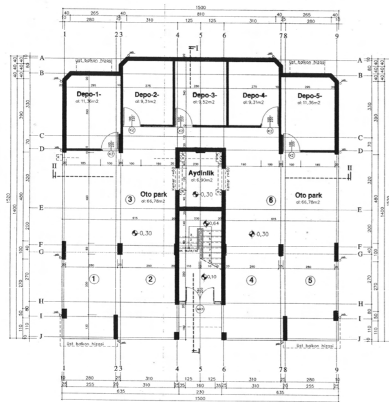
ZEMİN KAT ölçek:1/50 Brüt alan: 213.25m 2
