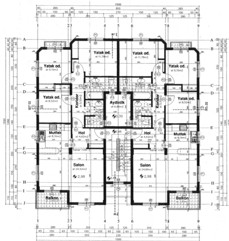
I. ve II. KAT PLANI ölçek:1/50 Brüt alan: 213.25m 2
